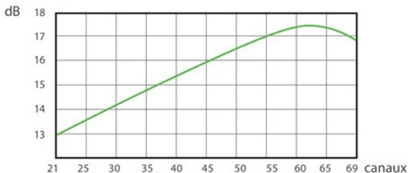
Diagramme de Gain
